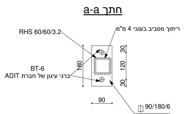
חתך עקרוני דרך המחיצות באיזור מזגנים
