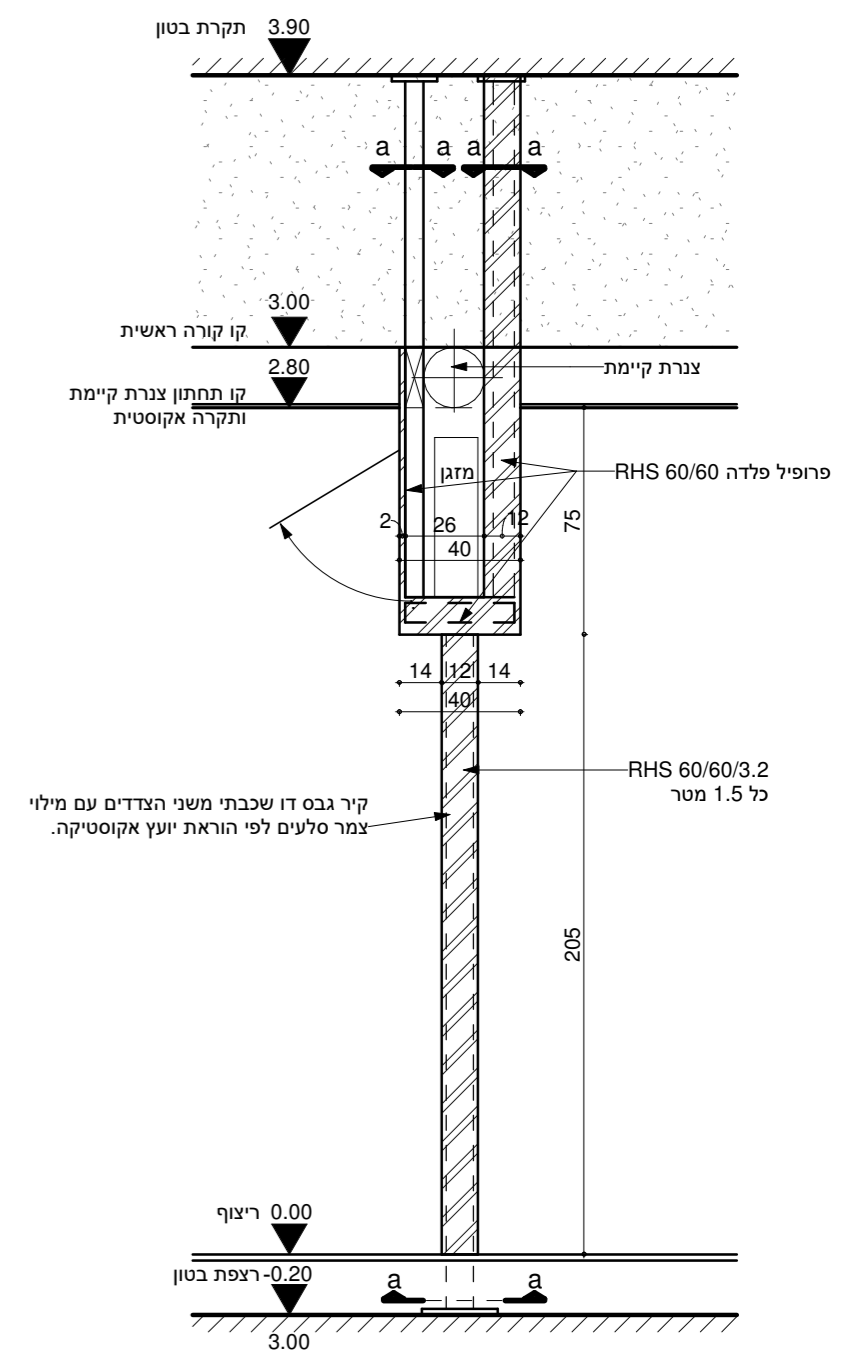
חתך עקרוני דרך המחיצות באיזור מזגנים
